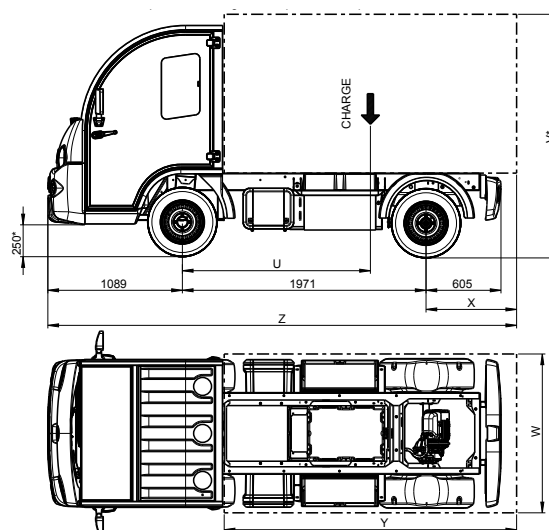
CHÂSSIS LONG
