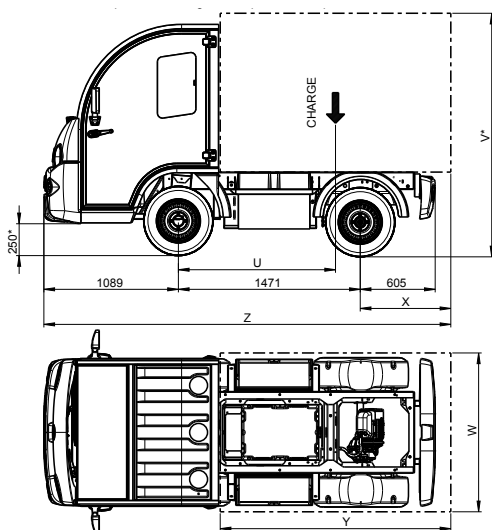
CHÂSSIS COURT
